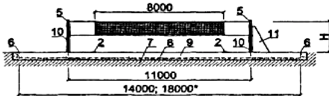
ПОПЕРЕЧНЫЙ РАЗРЕЗ
